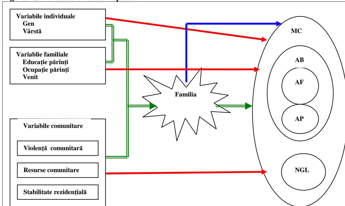
Figura 1 Schema teoretico-conceptuală
