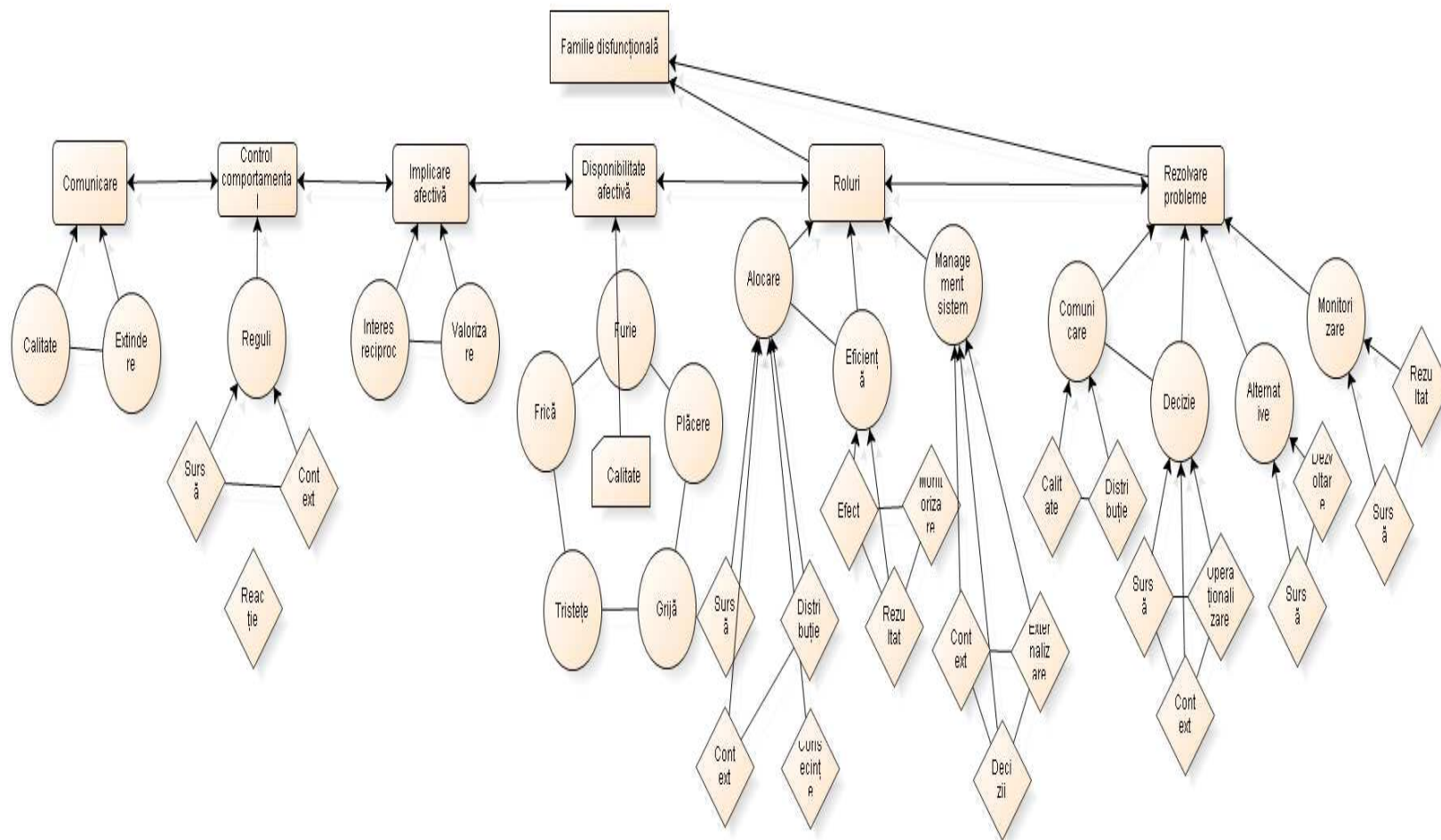
Figura 3 Schema categorică
